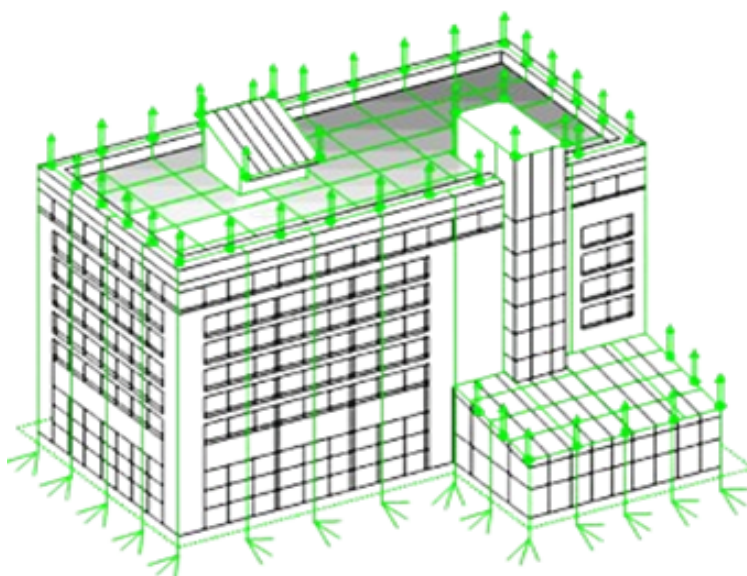
Visual System Faraday (Sangkar Konduktor)
